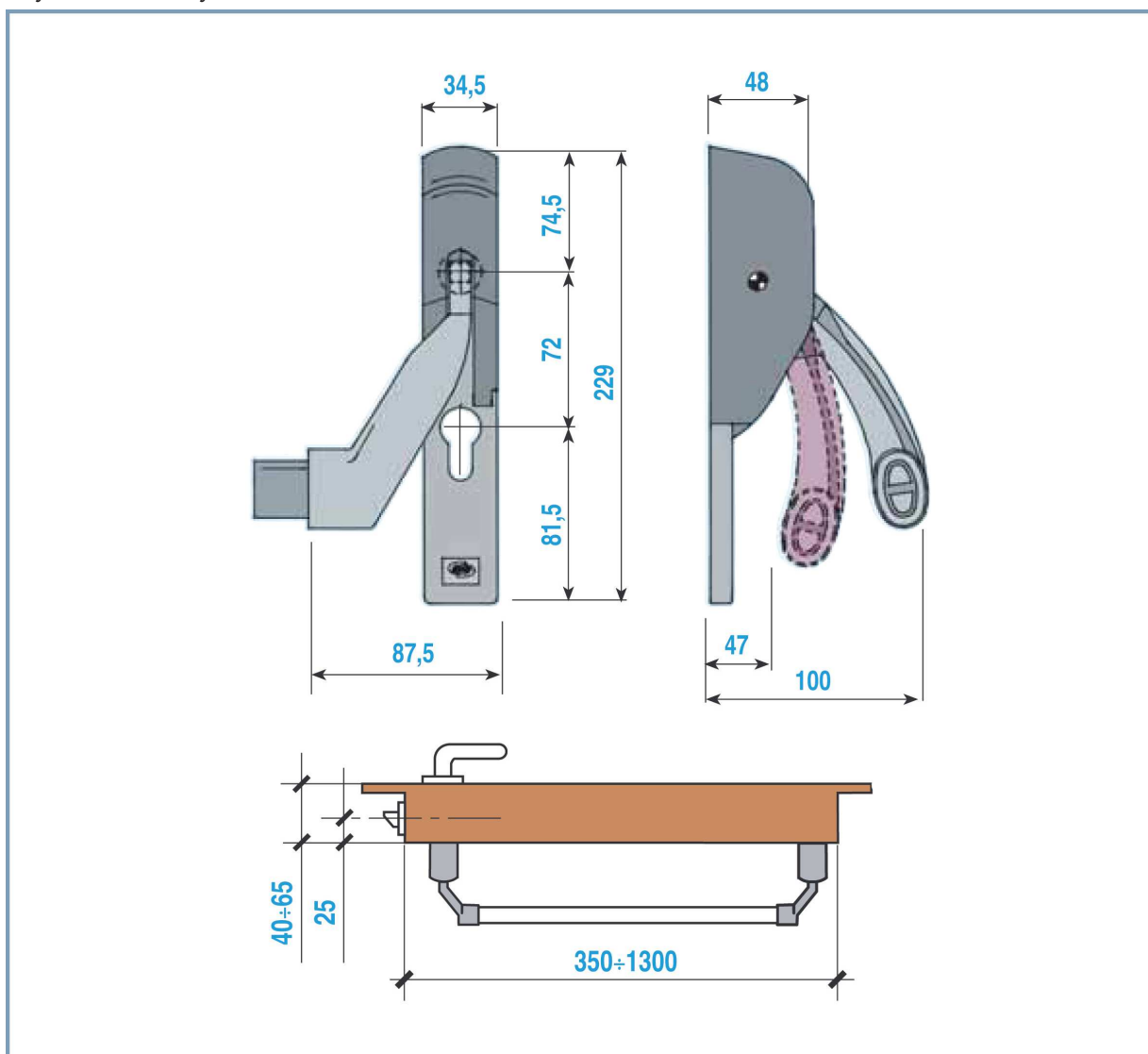
Rys. Techniczny
